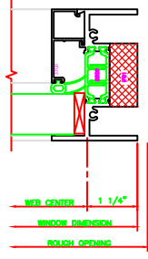
401 JAMB 325 FIXED
